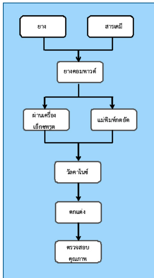
รูปที่ 2 กระบวนการผลิตชิ้นส่วนยางต่างๆ ที่ใช้ในรถยนต์
