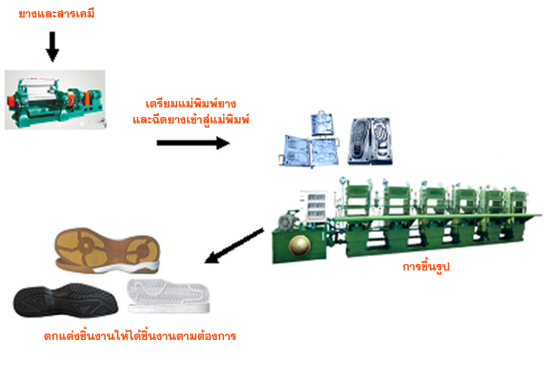
รูปที่ 1 กระบวนการผลิตพื้นรองเท้า
